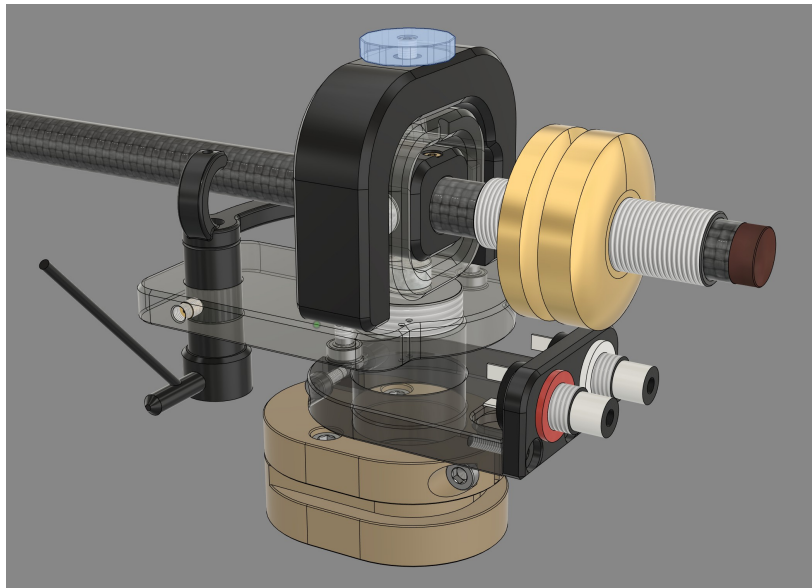
Bild 9: die Antiskatingschraube
